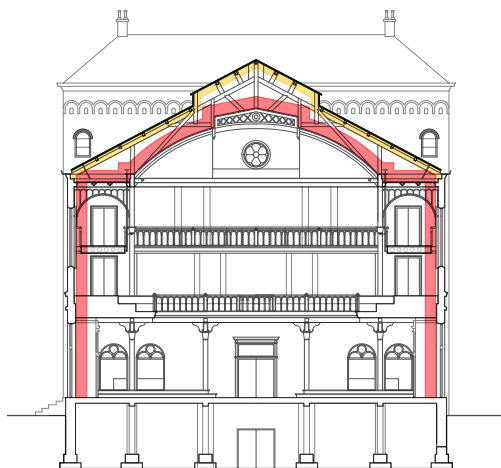
03 DAK VERZWAREN EN VOORZETWANDEN (600MM)
