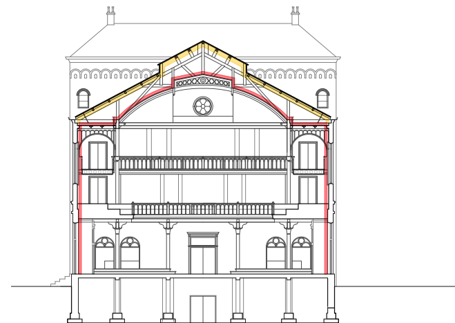
02 DAK VERZWAREN + ISOLEREN EN VOORZETWANDEN (200MM)
